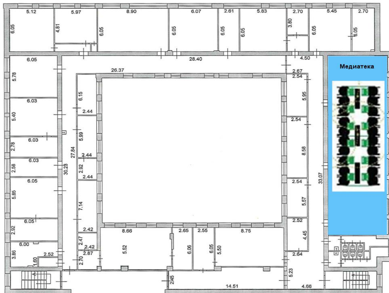
Рисунок 4. Зонирование помещений центра непрерывного повышения
